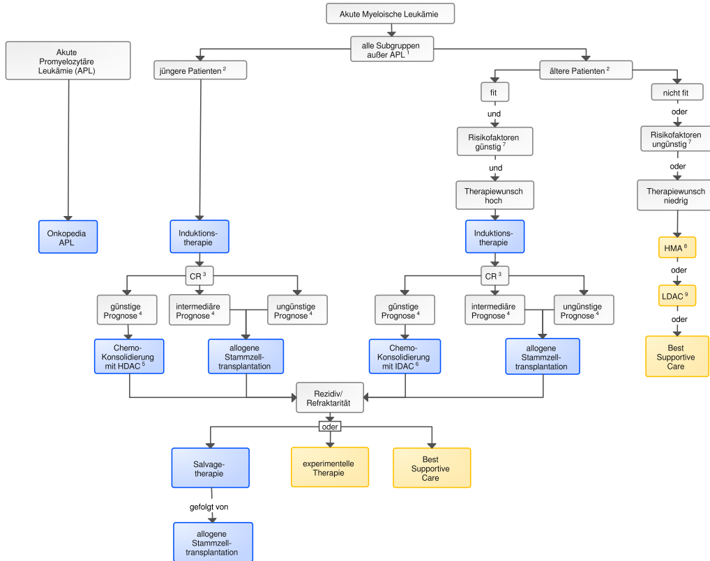
Abbildung 1: Therapie - Algorithmus
